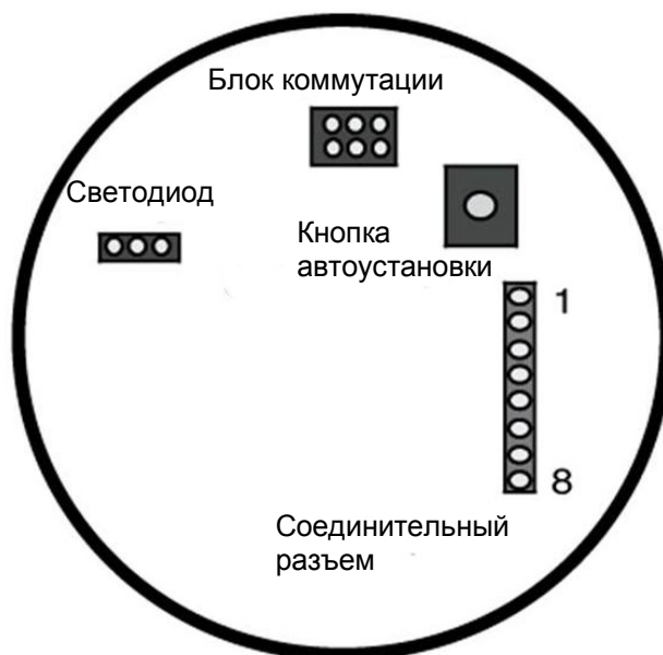
Рис. 4. Панель сенсора
